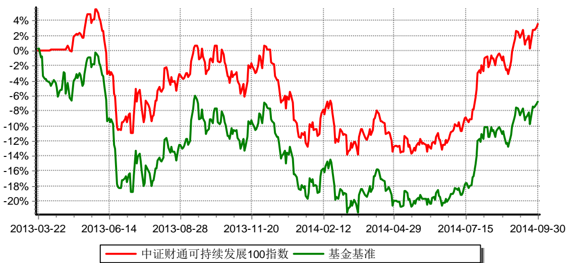
中证财通中国可持续发展100 (ECPI ESG) 指数增强型证券投资基金 累计净值增长率与业绩比较基准收益率历史走势对比图 (2013年3月22日-2014年9月30日)
